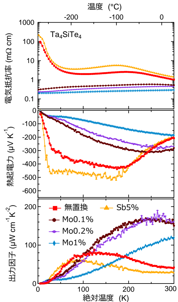
図2. 新材料 Ta_4SiTe_4 の熱電特性. 上から順に, 電気抵抗率, 熱起電力, 出力因子. 元素の添加を行っていない無置換試料と, MoまたはSb添加試料のデータを記載した.
