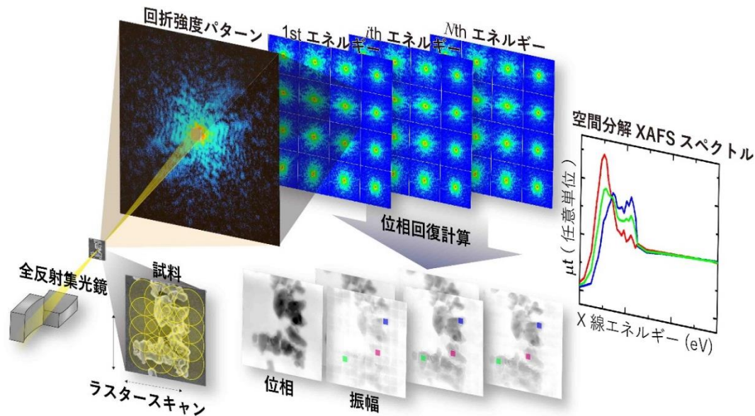
図 1 タイコグラフィ-XAFS 法の概念図
