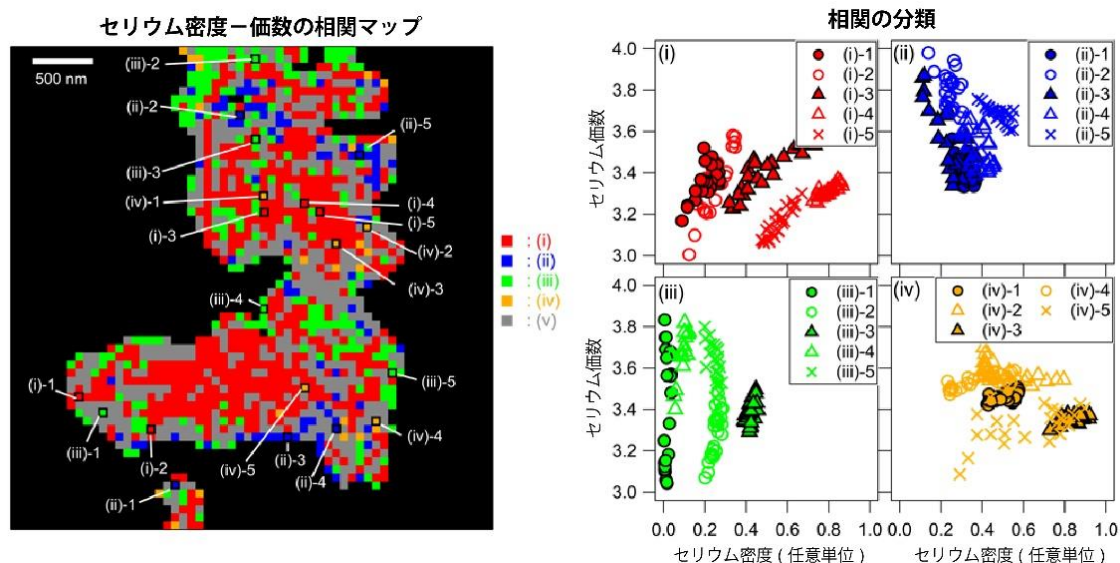
図 3 Pt/CZ-7.6 のセリウムの密度と価数の相関解析の結果
