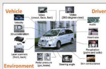
車両走行時のデータを収集するためのセンサ車両 Sensor-car for collecting run-time data
