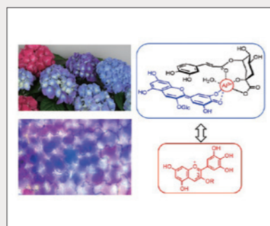
アジサイの花弁変色の本質は細胞毎に色が異なることにより、超分子錯体の形成に基づく複雑系現象の一つである。 Color change of hydrangea is a phenomenon of complex system due to the formation of blue supramolecule.
