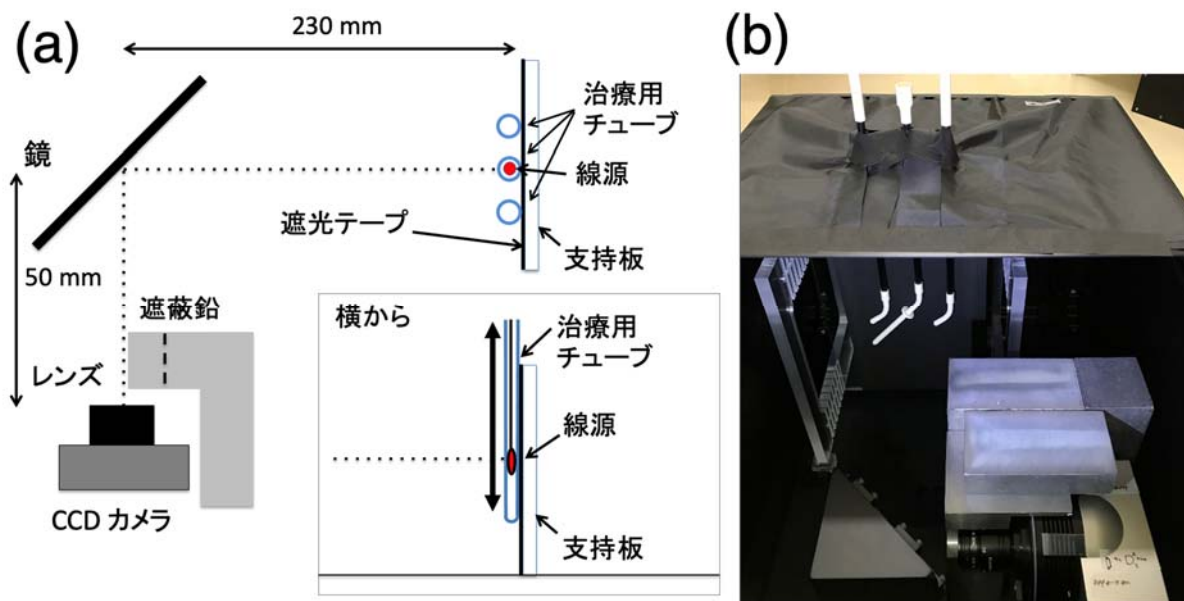
図2. 測定装置の概念図(a)と写真 (b)
