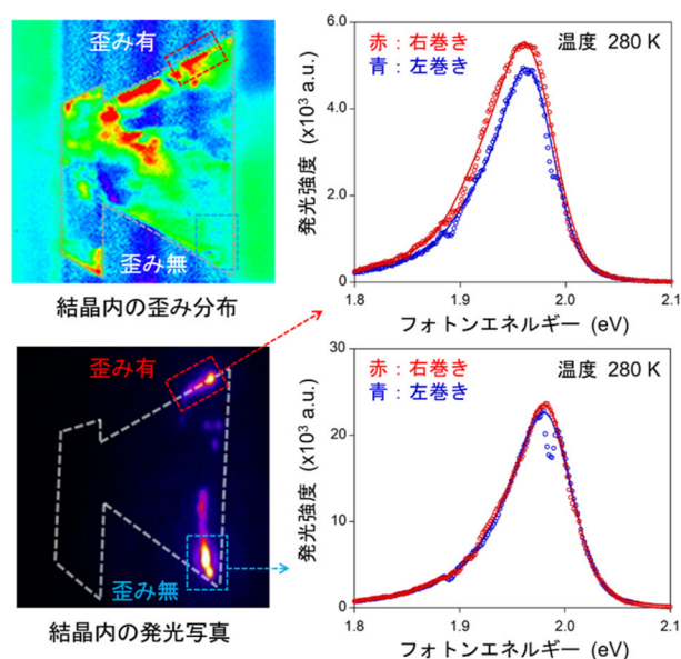
図2 結晶内の局所歪みに由来した強固な円偏光発光(ELスペクトル)
