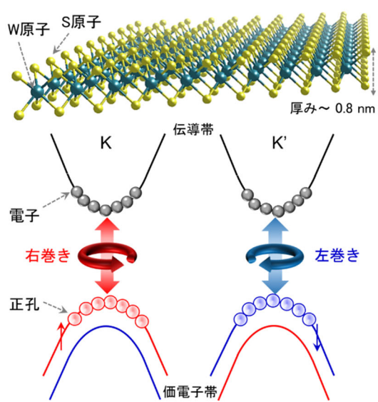
図1 単層TMDCの構造（上）とバレー分極（下）
