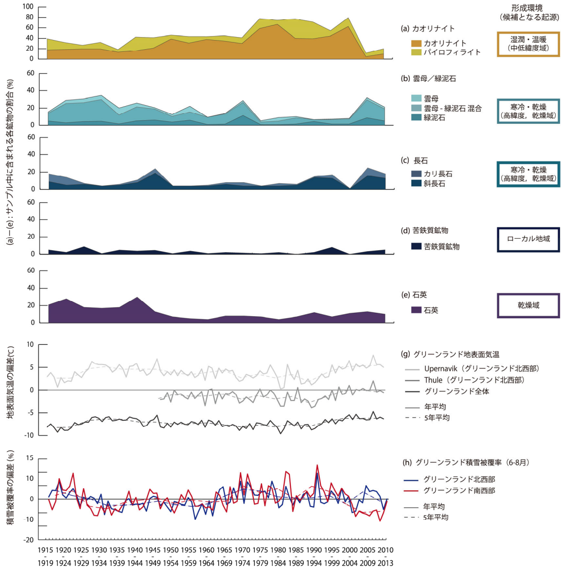
図4：タイプ別のケイ酸塩鉱物組成 (a-e) の変動と、グリーンランドの地表面気温 (f)、および積雪被覆率 (g) の偏差の変動を比較した結果。(g)のグリーンランド全体の気温は米国 Berkeley Earth, Upernavik と Thule (グリーンランド中西部, および北西部の町) の気温は Cappelen (2019) (文献1) の結果を引用。
