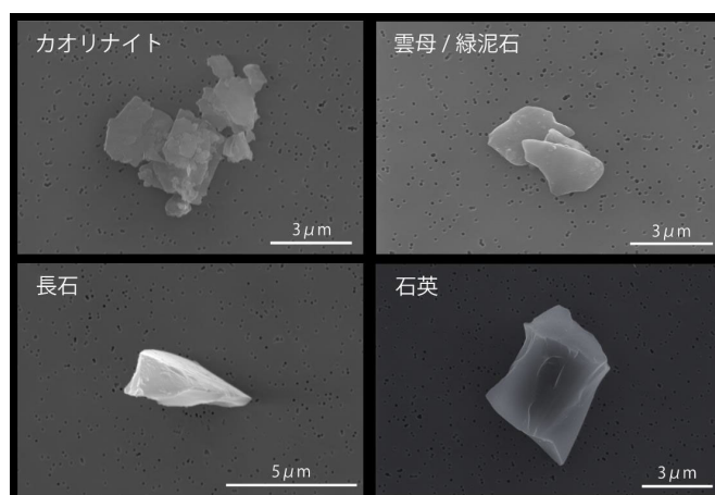
図 1： SIGMA-D アイスコアに含まれる鉱物ダストのうち、ケイ酸塩鉱物の SEM 画像。多数の黒い丸はフィルターの子。
