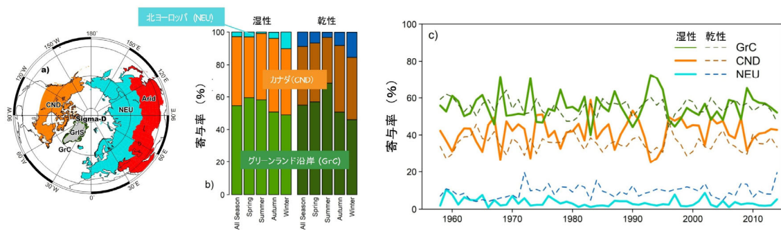
図5：(a) SIGMA-D サイトへの大気塊の寄与の可能性のある4つの地域 (GrC (緑)：グリーンランド沿岸部露岩域, CND (オレンジ)：カナダおよびアラスカ, NEU (青)：北ヨーロッパ, Arid (赤)：中国, 中央アジア, 中東の乾燥域)。湿性沈着および乾性沈着 (注2) を通じた各起源地域から SIGMA-D サイトへの大気寄与率の (b) 季節変動および (c) 年変動 (1958-2013年、氷床と海洋からの寄与は除く)。
