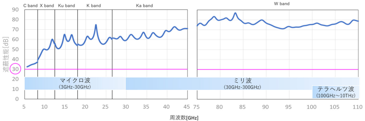
グラフ 1 新材料の電磁波遮蔽効果
