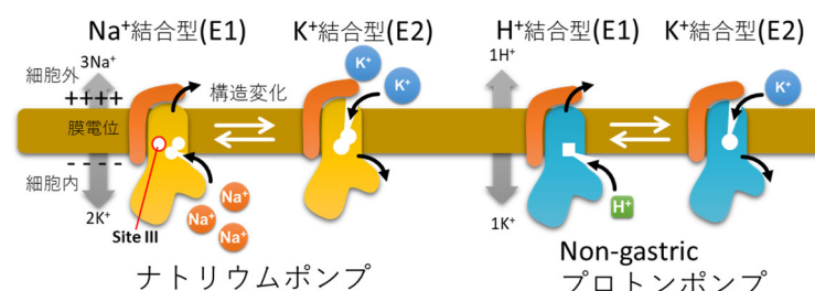
図 3 輸送イオンの違い
