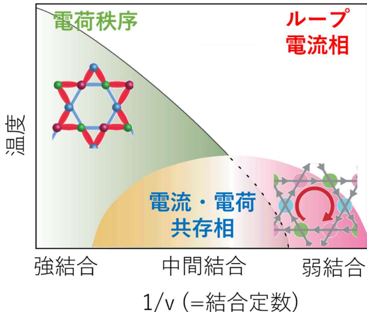
図 3 本理論で得られたカゴメ格子金属の状態相図。中間結合領域では、ループ電流秩序と電荷秩序が共存する。
