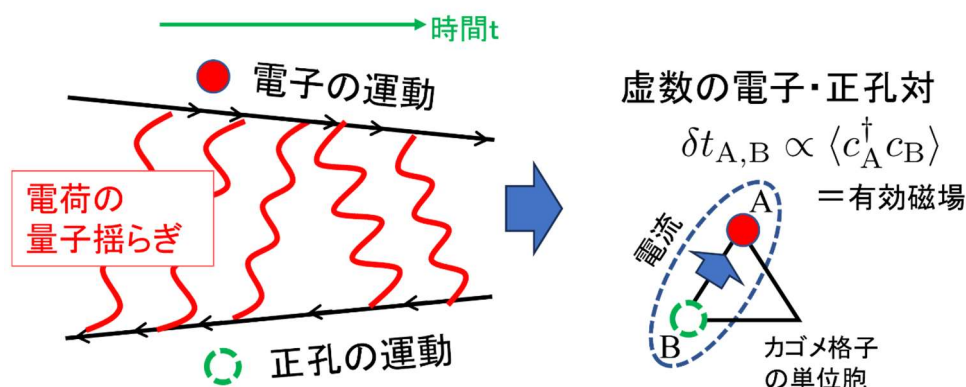
図 2 本研究で見出した“電荷揺らぎ交換電流秩序機構”の量子力学的過程(ファイマン図形)。本機構で導かれる虚数の電子・正孔対 \delta t は、自由電子に対する有効磁場を与えるため、減衰しない永久ループ電流が生じる。
