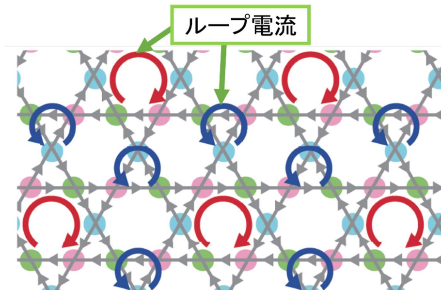
図 1 カゴメ格子金属における永久ループ電流。矢印が電流の向きを表す。ホールデンが予言したチャーン絶縁体の金属版である。自由電子がトポロジカルな有効電場を感じる結果、ナノスケールのループ電流が流れる。
