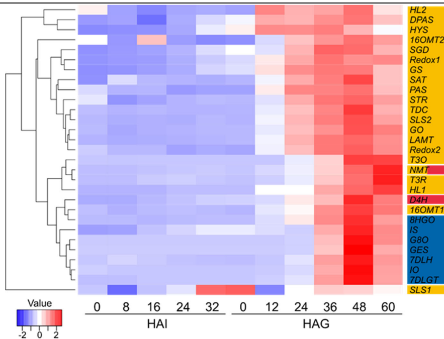
図2 アルカロイド合成酵素遺伝子の種子吸水・発芽に伴う発現変動
