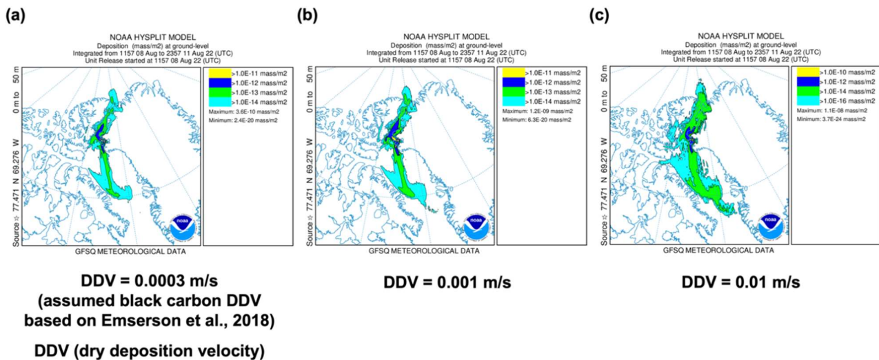
図 3. NOAA HYSPLIT モデルを用いた、三つの異なる乾性沈着速度 (DDV) によるカナックのゴミ置き場の地点からの粒子拡散による相対累積沈着量の計算：(a) DDV = 0.0003 \text{ m s}^{-1} (Emerson et al., (2018, doi: 10.1029/2018JD028954) によるブラックカーボンを想定した乾性沈着速度に基づく)；(b) DDV = 0.001 \text{ m s}^{-1} ；(c) DDV = 0.01 \text{ m s}^{-1} 。3.5 日間の前方拡散計算は、2022 年 8 月 8 日 11 時 57 分 (UTC) に開始した (図 2a の現地時間 9 時 57 分に基づく)。
