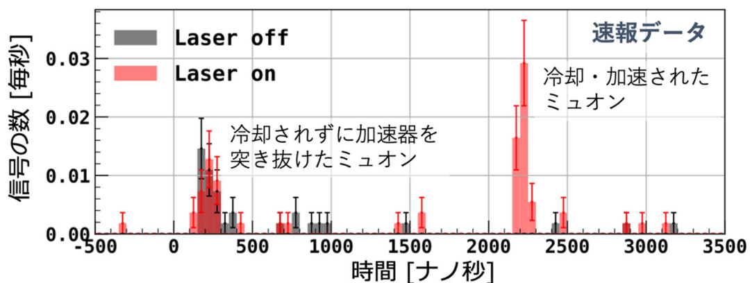
図 3 加速空洞出口で測定した粒子の時間分布と冷却・加速されたミュオンの信号。あらかじめ加速後に想定されるエネルギー（90 keV）と運動量を持つ粒子だけを選択し、測定している。
