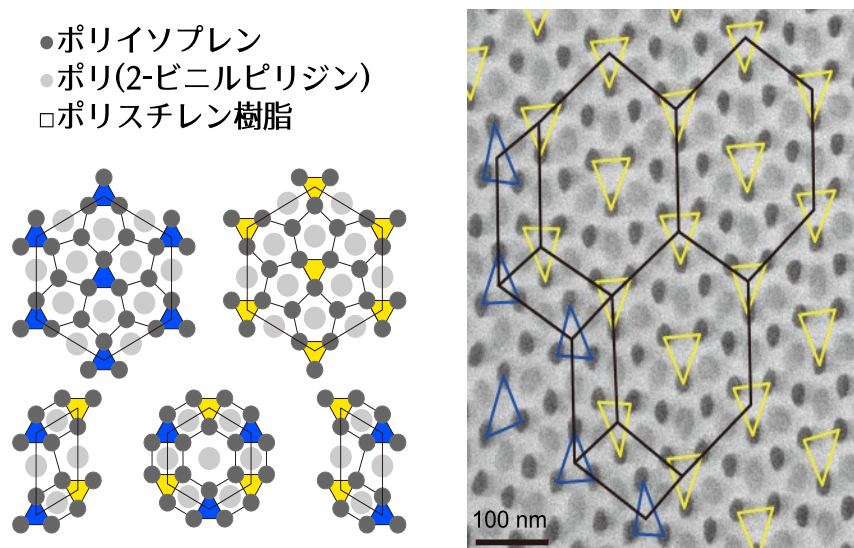
図 4. 複合高分子系の電子顕微鏡写真。黒丸はポリイソプレン、灰色丸はポリ(2-ビニルピリジン)を示す。これらの分子の間の白色の領域はポリスチレン樹脂によって占められている。
