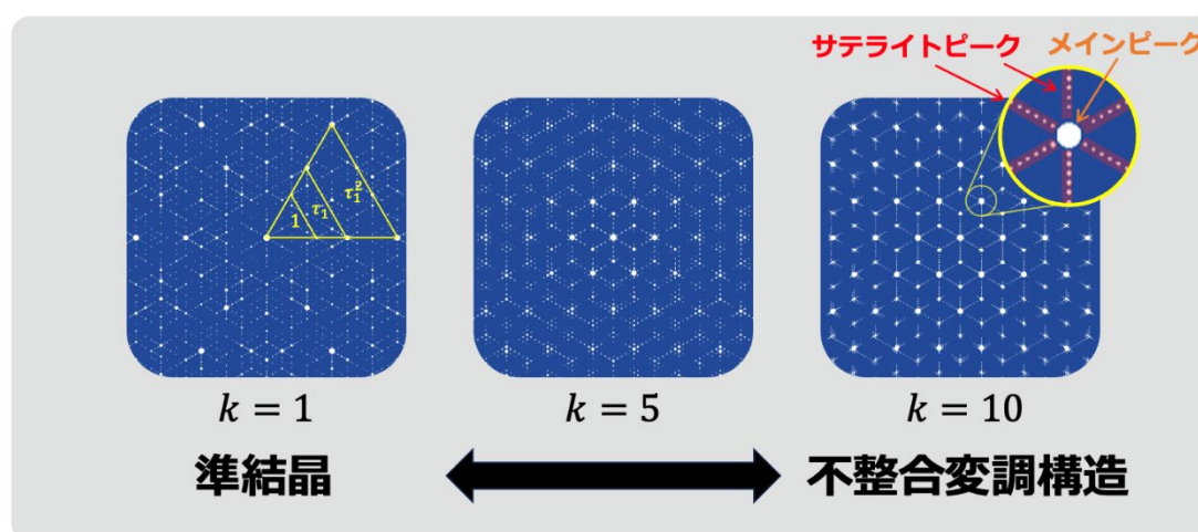
図 2. 6 回対称貴金属比準結晶の回折パターン
