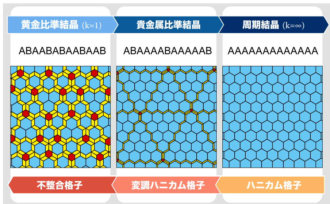
図 1. 6 回対称貴金属比準結晶タイリング。貴金属比の発散極限において、ハニカム格子に収束する。黄色で示される平行四辺形がドメインウォールを成している。
