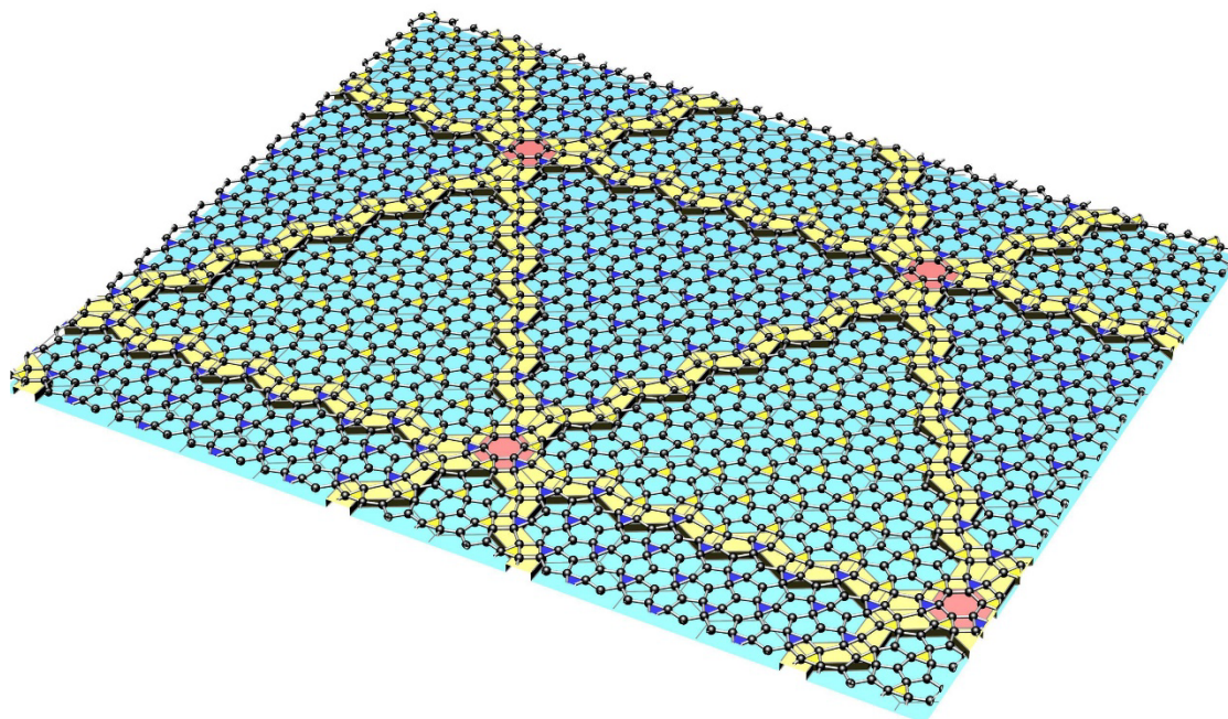
図 3. 不整合変調構造を有する分子配列と 6 回対称貴金属比準結晶タイリングの関係。青色と黄色の三角形は三角ドメインの異なる向きに対応している。
