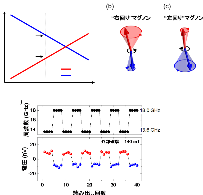
図 2 (a)垂直磁化の人工反強磁性体におけるマグノンの外部磁場に対する共鳴周波数。(b)右回りマグノンおよび(c)左回りマグノンの模式図。(d)特定の外部磁場下における伝播マグノンの回転極性制御の例。マイクロ波の励起周波数の切り替えに対応して、伝播したマグノンの検出電圧の符号が変化しており、伝播マグノンの回転方向を電氣的に読み取ることに成功しました。
