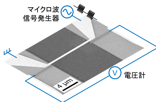
図1 本研究で作製したデバイスの電子顕微鏡図および測定回路の簡略図。
