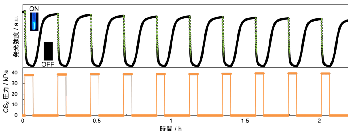
図 4. \text{CS}_2 吸着/脱着プロセス中の in situ (その場) 発光測定の結果。オレンジのグラフ (下側) は \text{CS}_2 の圧力、黄緑色のグラフ (上側) は MOF の発光強度を示しており、 \text{CS}_2 圧力の増減 (吸着/脱着) 処理に対応して発光強度の ON-OFF が 10 サイクルに渡って可逆的に起こることから優れたリサイクル性を実証しました。
