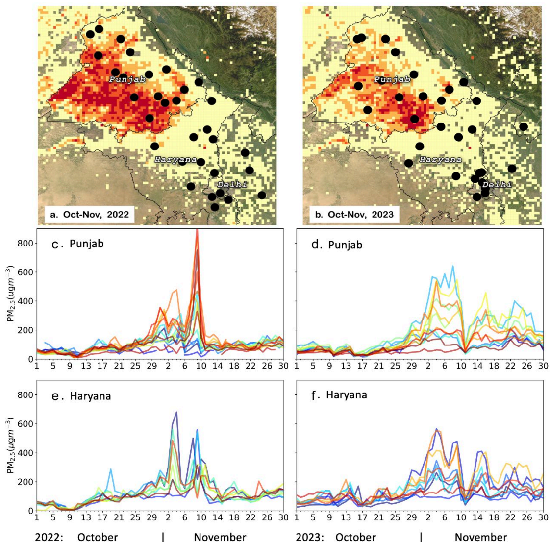
図 1. 上段の図は、NASA の人工衛星 SNPP および NOAA20 衛星に搭載された可視近赤外放射計群 (VIIRS)による緯度経度 0.05 \times 0.05 度 (約 5 km) の解像度の火災検知数分布を示し、背景に地表面の可視画像を示しています。図 a, b の黒い丸の地点には約 30 台の計測器 CUPI-G を設置しています。コメなど夏作物が収穫された直後の 10 月下旬から 11 月にかけて、インド北西部で衛星から多数の農地火災が検出されました(a:2022 年, b:2023 年)。下段の図は、パンジャブ州(c, d)、ハリヤーナー州(e, f)に設置したすべての CUPI-G から得られた PM_{2.5} 濃度の時間変化です。観測結果から、パンジャブ州(c, d)とハリヤーナー州(e, f)の農村部の PM_{2.5} による大気汚染は、2022 年(左列)と 2023 年(右列)のどちらも、10 月から 11 月にかけての農業残渣焼却によって悪化することがわかりました。
