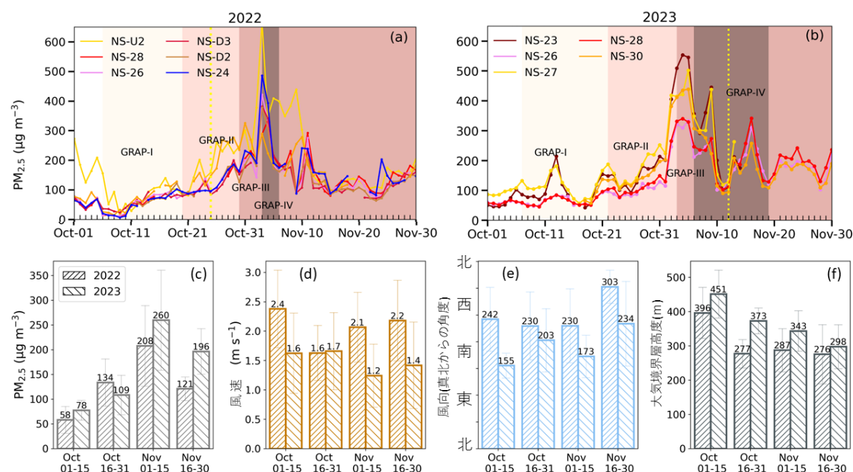
図 2. 大都市デリーとその周辺地域における \text{PM}_{2.5} 濃度は、主にデリー地域内での排出が支配的で、デリー首都圏の発生源に焦点を当てた GRAP 規制の実施によってコントロールされて
