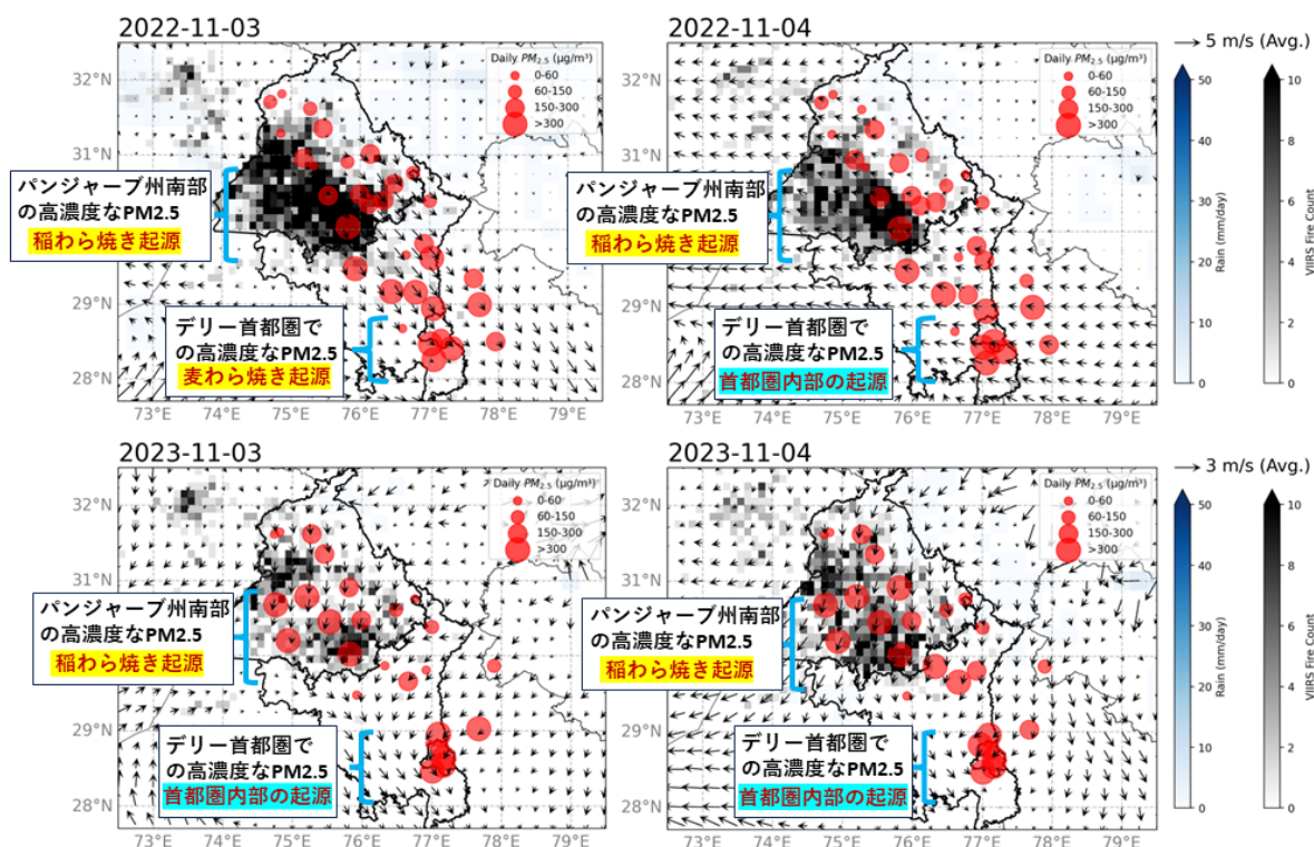
図 3. Aakash/CUPI-G の地上観測ネットワークにより、パンジャブ州からデリーまでの空気の動きを可視化した図です。デリー首都圏で高濃度の PM 2.5 が観測された 4 日間(2022 年;上段、2023 年;下段)を示しています。農業残渣焼却によってパンジャブ州南部の日平均 PM 2.5 濃度(赤い丸)は常に上昇しますが、その直接的な影響がデリー首都圏に到達することはめっ
