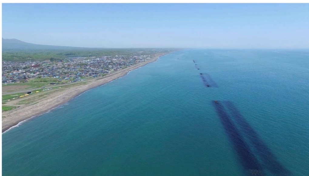
図 1. 白老沖のタンデム型人工リーフ（空中写真、撮影巻口範人）
