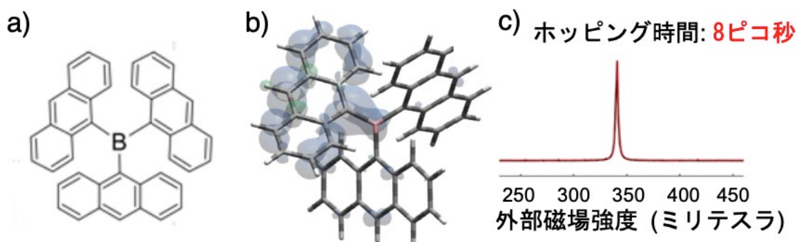
図1. a) 本研究で使用了光アップコンバージョンを行う三量体発光体分子:トリ (9-アントリル) ボラン (TAB) の構造式。b) 三重項-三重項消滅(TTA)を行う中間体立体構造と、その励起子が持っている二つの電子スピン密度分布画像。c) オクタエチルポルフィリン (PtOEP) を増感剤として用いたトルエン-流動パラフィン混合溶液において得られた TAB 三重項励起子の時間分解電子スピン共鳴スペクトル。図2によるモデル解析によって、分子内において三重項励起子ホッピングが8ピコ秒(1兆分の8秒)の時間で進行することが分かった。
