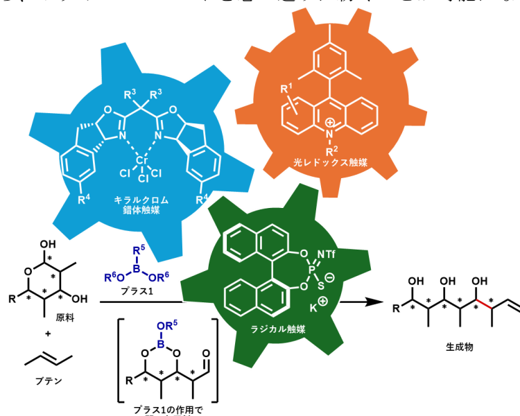
図 2：今回開発した触媒システム
