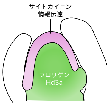
図 4 メリステムにおけるフロリゲンとサイトカイニン情報伝達の空間的分布。
