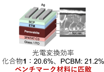
図 3 本研究で開発した新規電子輸送材料の合成、構造、ならびに素子特性
