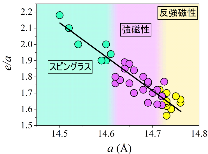
図3 Tsai型化合物における磁気相図。Tsai型化合物の磁気状態を格子定数と価電子濃度（ e/a ）の関係で整理した結果、スピングラス（Spin-glass）、強磁性（Ferromagnetic）、反強磁性（Antiferromagnetic）の各磁気状態が、化学組成や希土類元素の種類によらず、格子定数によって一つの磁気相図上に統一的に分類できることが明らかとなった。従来用いられてきた e/a では物質系によって磁気相境界が異なるのに対し、格子定数を用いると異なる物質系のデータが共通の相境界に集約される。本研究で得られた磁気相図は、新しい磁性準結晶や近似結晶、さらには未知の磁気秩序を示す新物質を探索するための実用的な指針となる。
