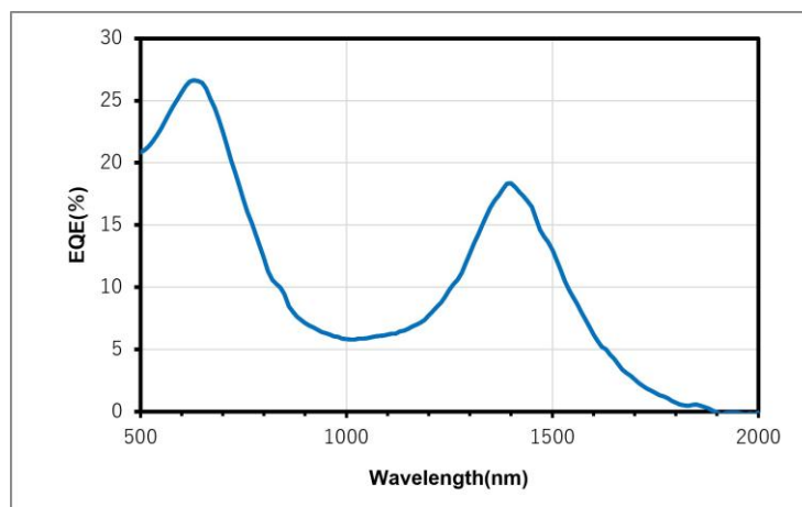
c) 可視～短波長赤外光をデバイスに照射した際の外部量子効率（EQE）の波長依存性
