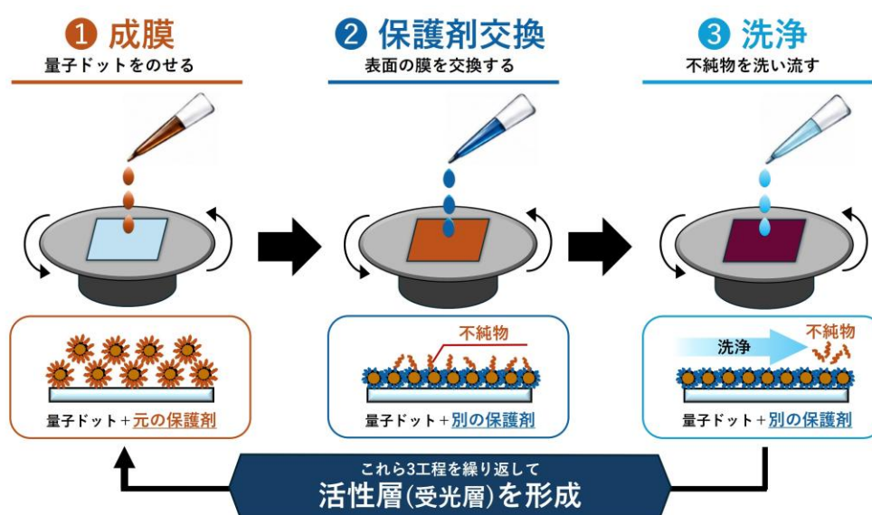
a) 印刷プロセスによるAg-S-Te活性層（受光層）の形成工程概略図
