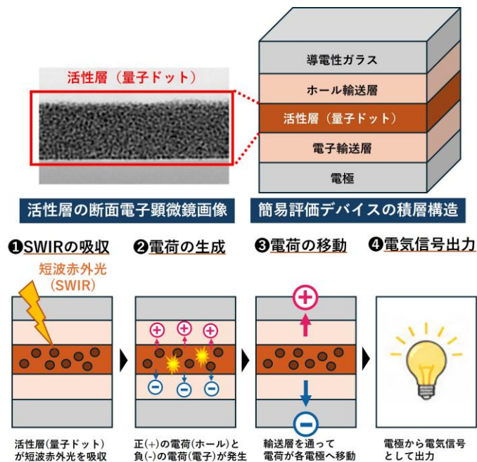
b) 積層した量子ドット材料の断面電子顕微鏡画像、簡易評価デバイスの積層構造
