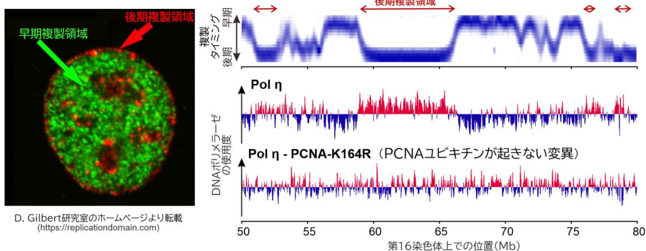
図2 後期複製領域における Pol \eta の合成バイアス
