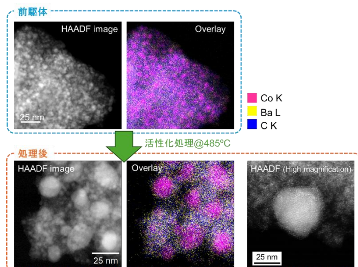
図3 収差補正 STEMによって観察した (\text{Ba}/\text{Co})_{0.3}/\text{C} 触媒の活性化処理前後の状態 EDS による元素マッピングからも活性化処理前の前駆体の内部には Ba と Co が微細な状態で分散していることがわかる。これを活性化(水素気流下、 485^{\circ}\text{C} )で処理することで、酸化 Ba の微細な粒子が Co ナノ粒子を覆った構造を炭素フレームの中に構築できた。
